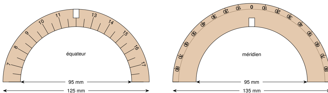
FIG. 2 – Les deux demi-couronnes du cadran solaire.
