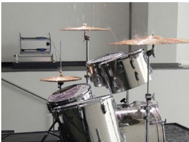
Fig.1. Exposée au Musée des Abattoirs de Toulouse en 2014, l'installation artistique «Averses» de Céleste Boursier-Mougenot matérialise la présence invisible des rayons cosmiques. Lorsque le télescope à muons (en arrière-plan à gauche de la batterie) détecte le passage d'une gerbe cosmique, une électrovanne d'une arrivée d'eau est actionnée. Située au plafond à environ 25 m au-dessus de l'instrument, celle-ci libère une courte mais intense averse d'eau. Les gouttes de cette douche font sonner les tambours et les cymbales, à des intervalles d'environ deux minutes en moyenne.
