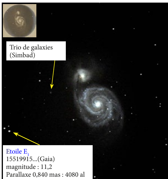
Fig.2. Image compositée de M51 au SCM 300 mm F/D=5, pour 40 poses de 30 secondes (20 min) à 1 600 ISO. Traitée par IRIS avec rehaussement dynamique et ajustement de contraste. Magnitude limite environ 18,2.
