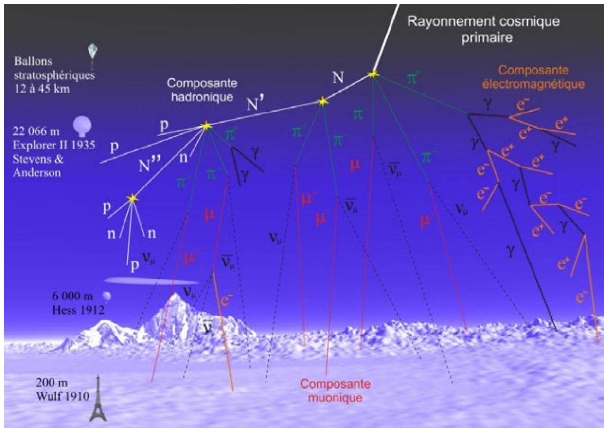
Formation de gerbe de particules par interaction des rayons cosmiques avec l'atmosphère (crédit C. Lagoute). Extrait du dossier pédagogique de Cosmos à l'école.
