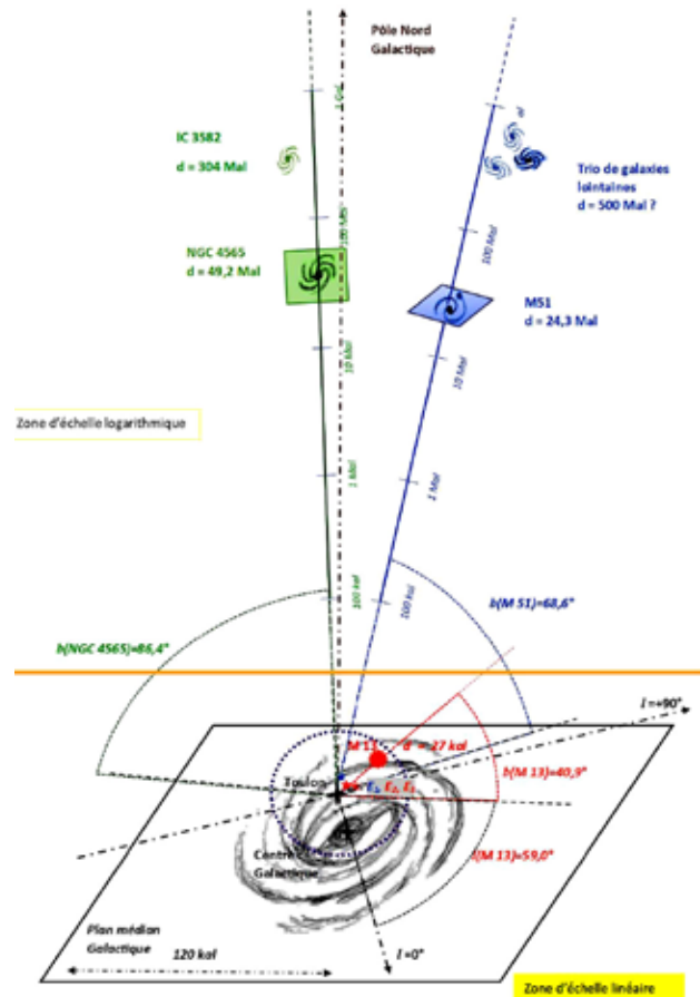
Fig.6. Vue récapitulative, en perspective. La partie supérieure est en échelle logarithmique. En réalité les diamètres des galaxies sont du même ordre de grandeur, y compris la Voie Lactée. Pour M51, son plan galactique est perpendiculaire à la direction d'observation. Pour NGC 4565, la plan de la galaxie contient l'axe de visée.
