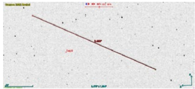
Fig.3. L'image de la figure 2 est téléchargée dans Aladin. Zoom sur la trace laissée par Cosmos 2022 Rocket ; Tag0 correspond à la position du zénith, dont les coordonnées ont été récupérées avec le logiciel Carte du Ciel à l'heure et au lieu de la photographie. L'outil de mesure des distances est utilisé sur la trace du satellite.
