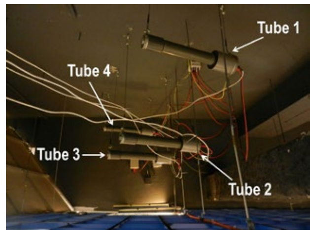
Fig.4. Disposition des détecteurs dans l'expérience « Effet est/ouest ».
