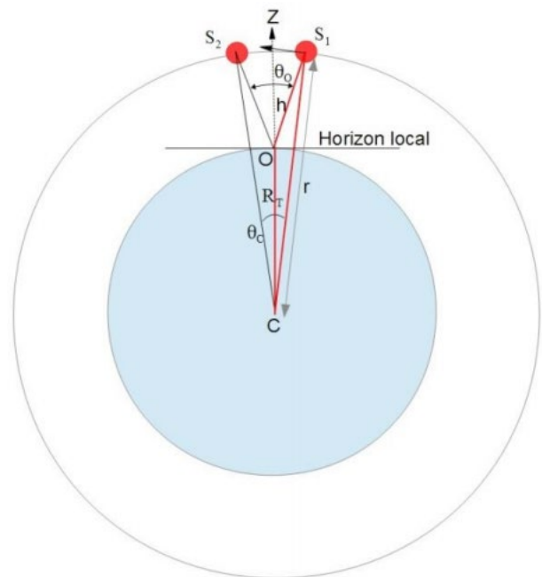
Fig.4. Modèle géométrique du phénomène observé. La figure est faite dans le plan de l'orbite du satellite. Ce plan contient l'observateur car le satellite passe au zénith. Source Pascal Descamps, IMCCE Observatoire de Paris.
