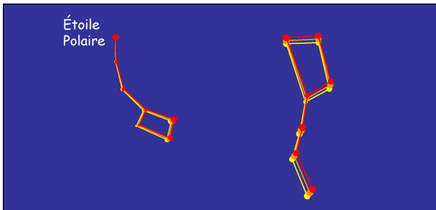
Fig.5. Petite Ourse et Grande Ourse représentées le 1 er décembre à minuit (en jaune), le 2 décembre à minuit (orange), le 3 décembre à minuit (rouge).
