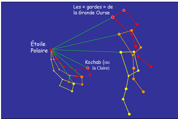
Fig.3. Petite Ourse et Grande Ourse représentées le 1 er décembre à 0 h (en jaune), 1 h (en orange) et 2 h (en rouge).
