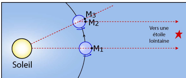
Fig.4. Mouvement relatif Terre/voûte céleste/Soleil sur un jour. En M 1 , il est minuit, un observateur voit une étoile. Après un jour sidéral (environ 23 h 56 min), il se retrouve en M 2 et voit l'étoile dans la même position. Mais il faut encore près de 4 minutes pour qu'il se retrouve à minuit en M 3 .
