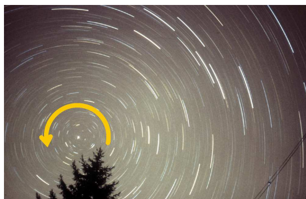
Fig.2. Mouvement relatif Terre/voûte céleste (pose photo d'une heure). L'étoile Polaire est au centre du mouvement apparent.
