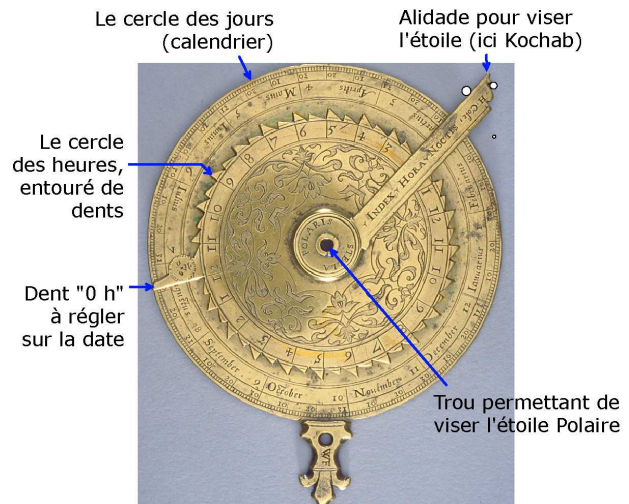
Fig.8. Les trois pièces du nocturlabe.
