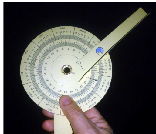
Fig.11. Nocturlabe proposé sur le site du CLEA. (www.clea-astro.eu, archive des Cahiers Clairaut, hiver 2013)
