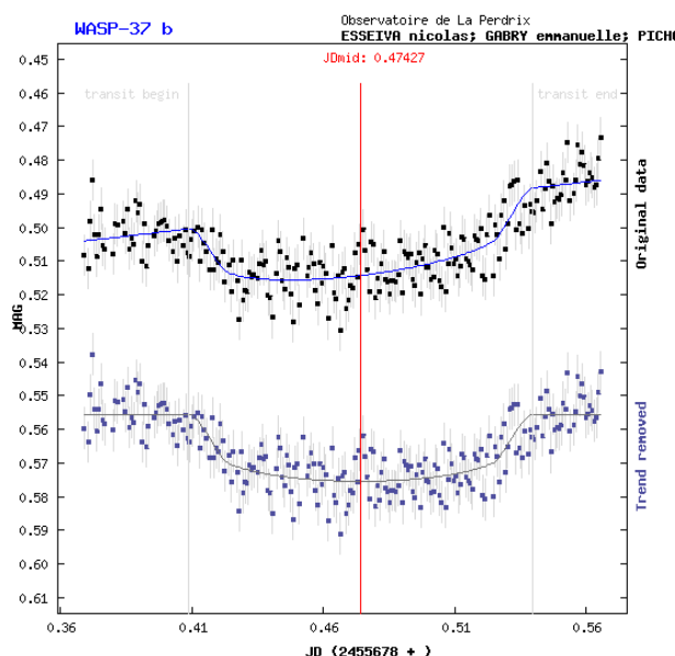
Fig.4. La courbe brute puis corrigée du transit de l'exoplanète Wasp 37b.
